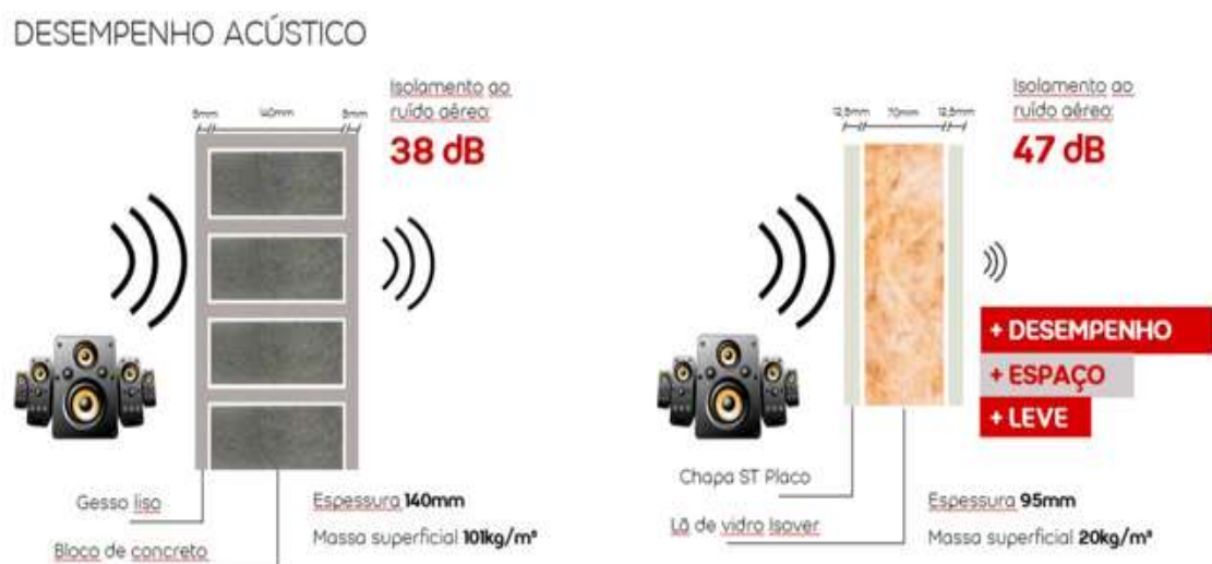
Figura 4 – Comparação acústica entre sistema LSF x convencional.
